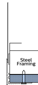
Drywall Trimless
